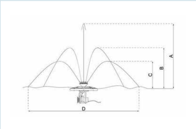
Fuente flotante con aireación máximo 6 focos.
